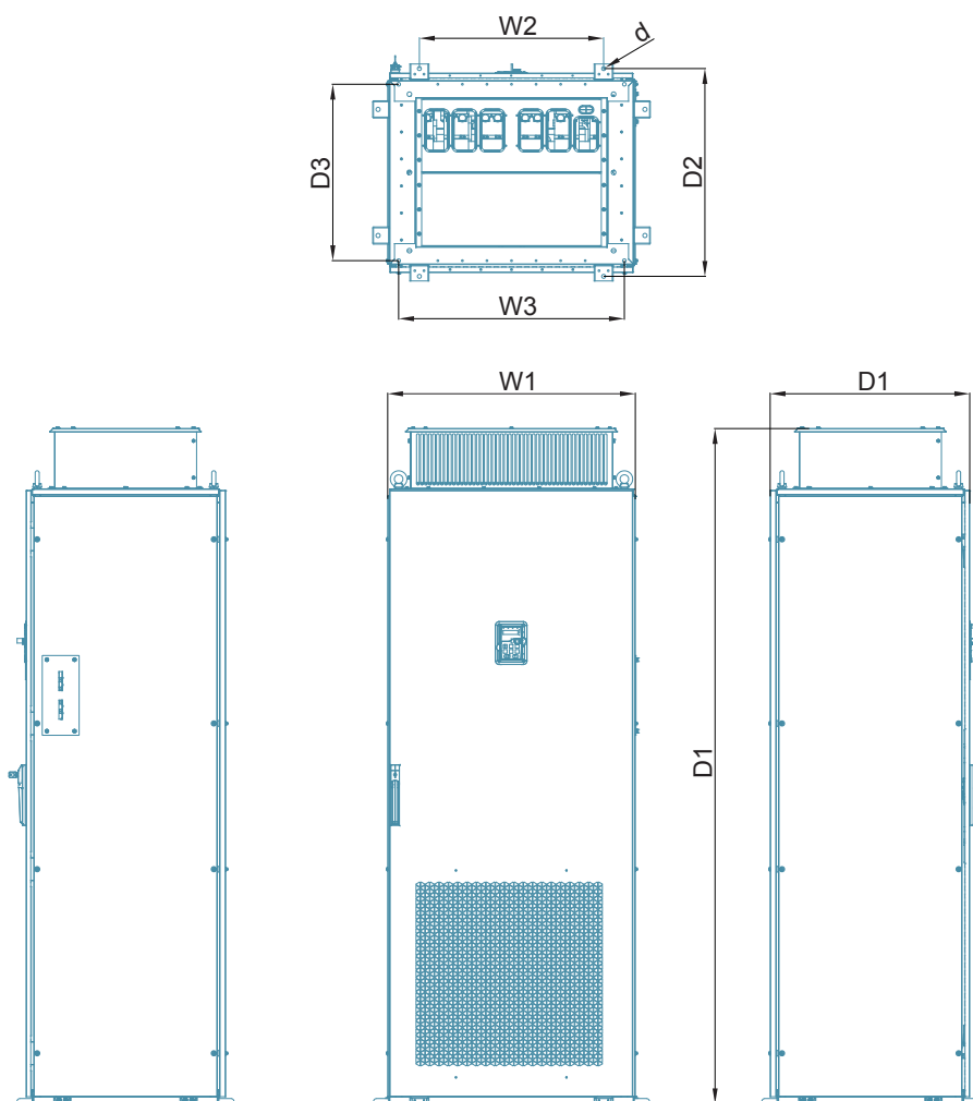
Чертеж для напольного монтажа моделей ПЧ 710–800 кВт
