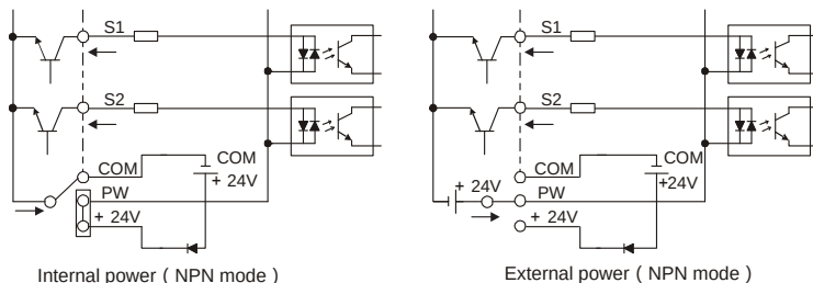
Рис. 4-36 Режим NPN
