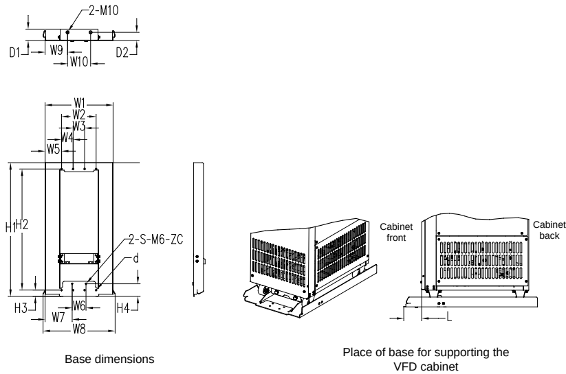
Рис. С-15 Размеры и монтаж монтажных кронштейнов для моделей 380 В 220–500 кВт
