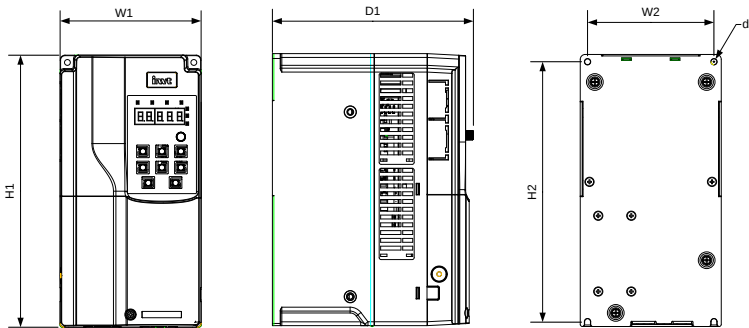
Рис. С-5 Чертеж для настенного монтажа моделей ПЧ 11–45 кВт
