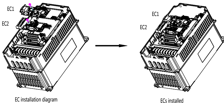
Рис. А-2 ПЧ с установленными платами расширения 11–500 кВт
