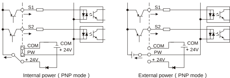
Рис. 4-37 Режим PNP415
