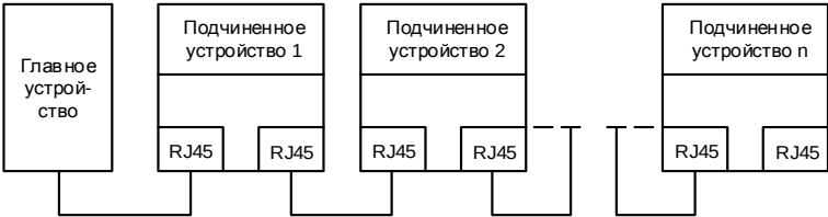
Фигура A-1 Схема электрических соединений топологии линейной сети
