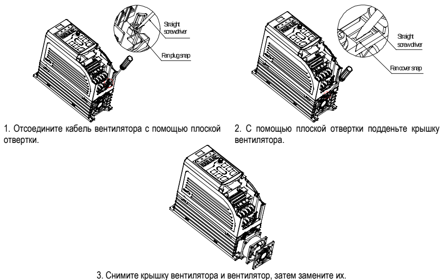
Рис.8-1 Обслуживание вентилятора для моделей 2,2–7,5 кВт (с помощью инструментов)
