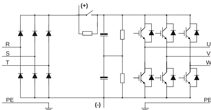
Рис. 3-1 Главная цепь
